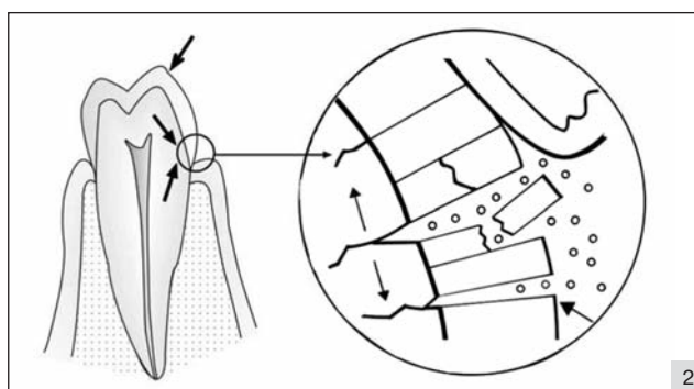
Рис. 2. Происходит выталкивание ионов кальция из кристаллической решетки гидроксилapatита эмалевых призм. Иллюстрация Lee and Eakle.
